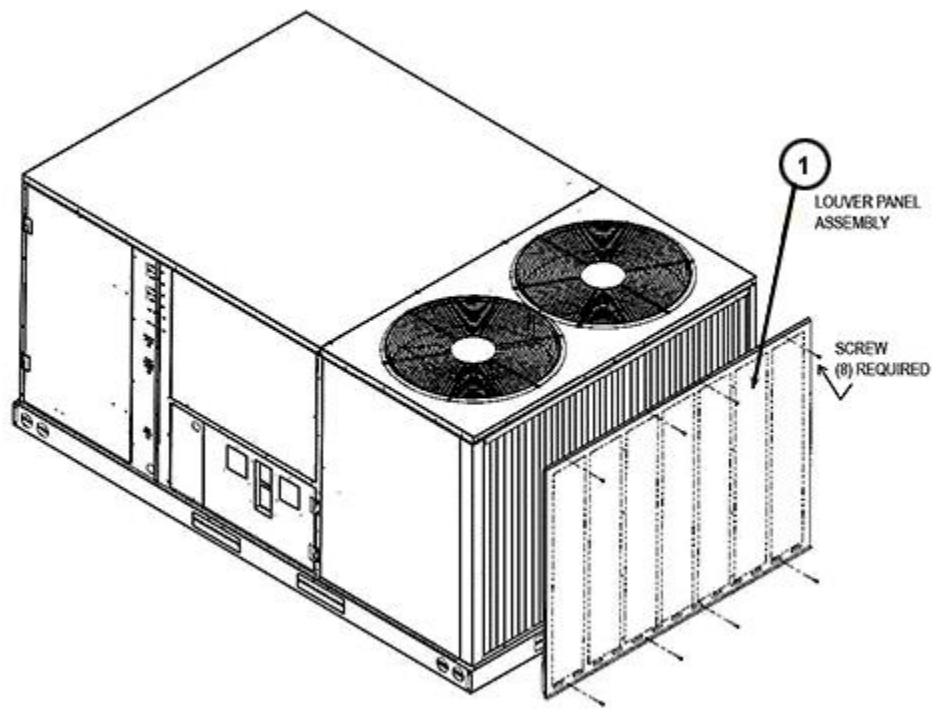
RXRX-AAD01C Assembly
