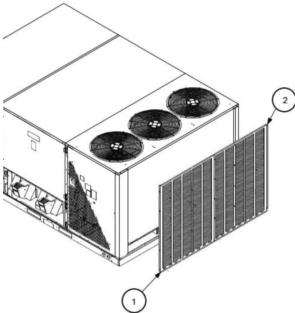
RXRX-AAD01K ASSEMBLY
