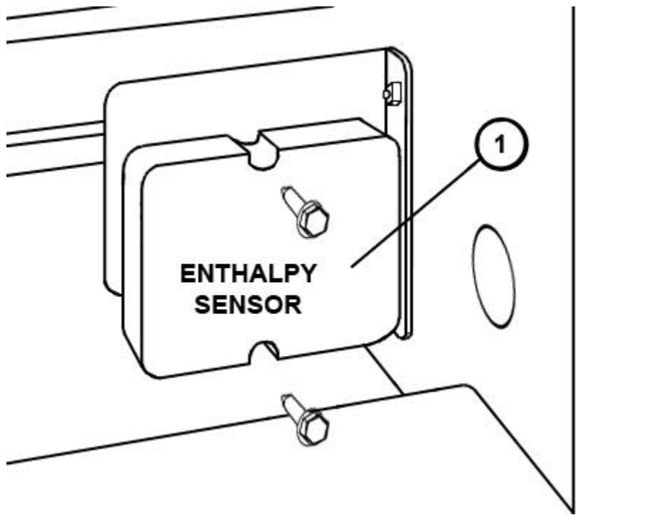
RXRX-AV02 Assembly
