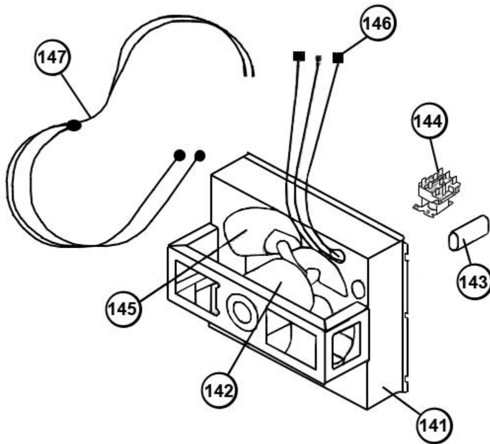
RXRX-BFF02x Assembly
