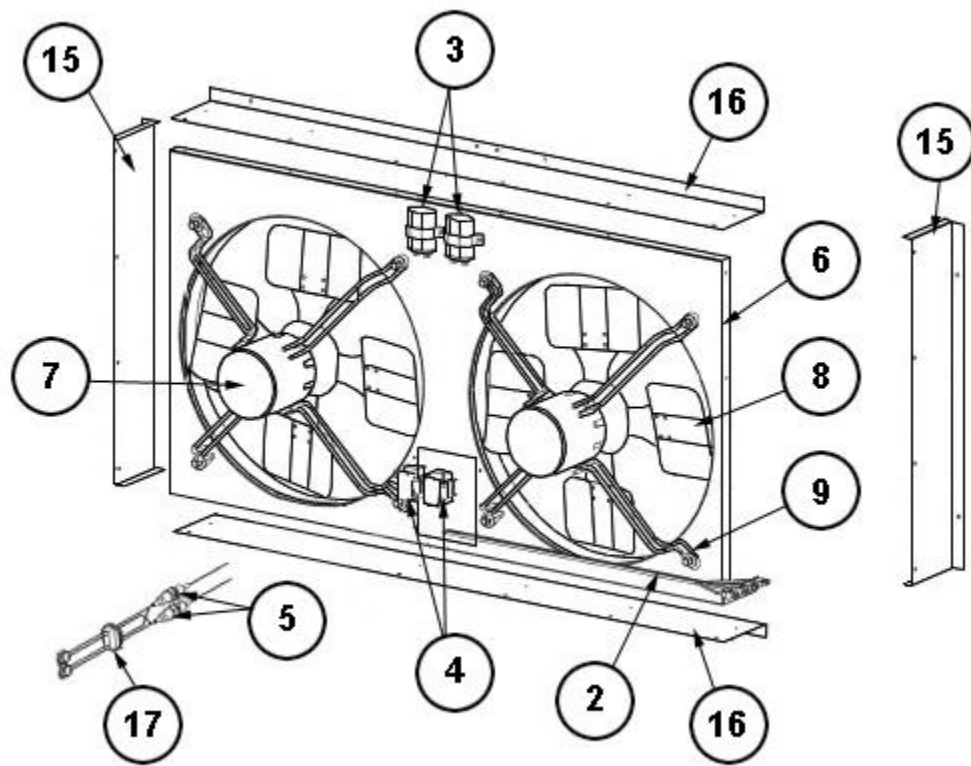
RXRX-BGF05 Assembly
