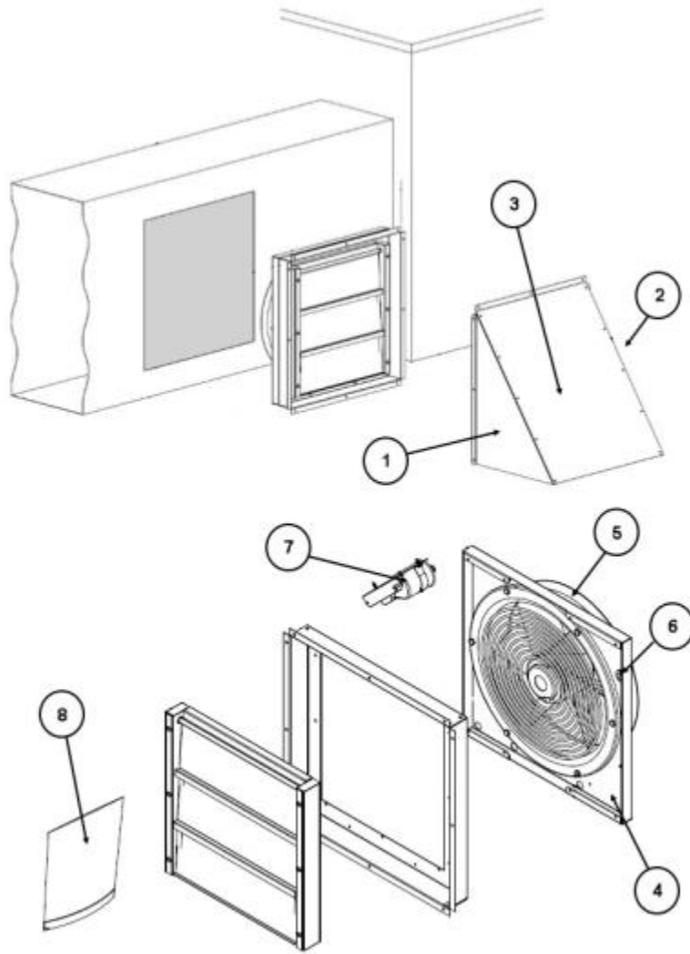
RXRX-CCF03C Assembly
